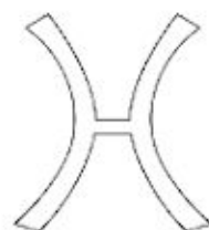
Pisces
