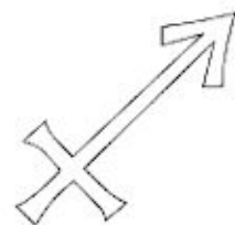
Sagittarius
